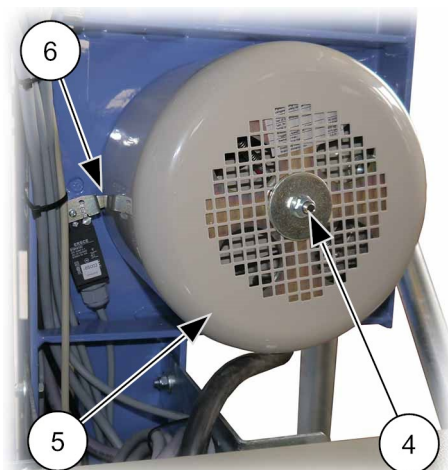
III. 70: Dispositif de freinage avec interrupteur de fin d'urgence
