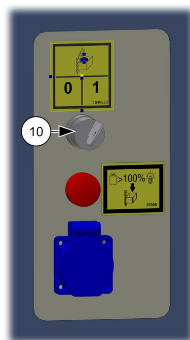
III. 48: Sélecteur Mode de fonctionnement Montage
