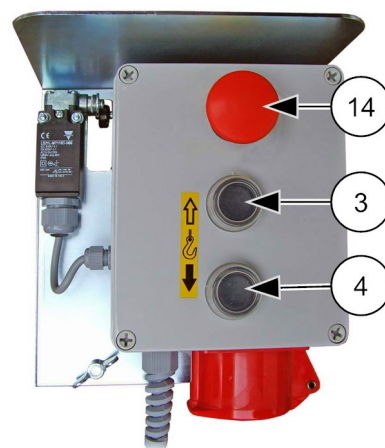
III. 46: Module électrique pour l'encagement d'accès sécurisé
