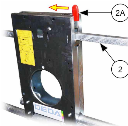
III. 40 – Ouverture / Fermeture de l'encagement d'accès sécurisé « Comfort »
