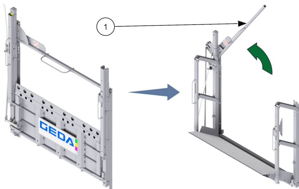
III. 32: Ouvrir/fermer la barrière avec verrouillage électromécanique
