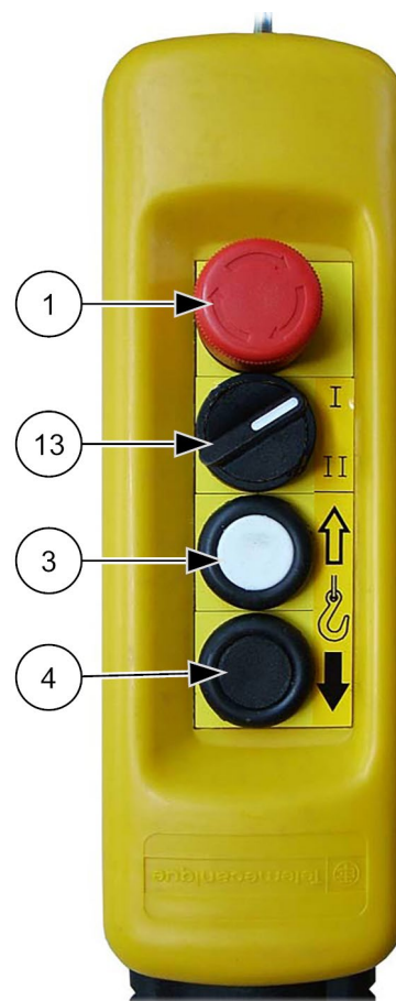
III. 42: Commande au sol / Commande manuelle (position I)
