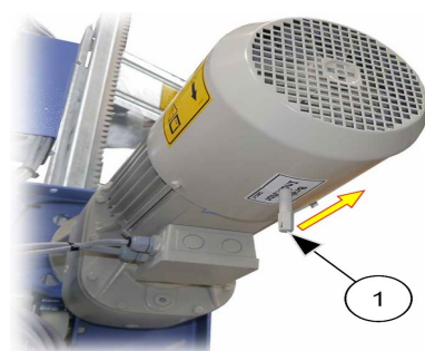
III. 73: Tirer le levier de desserrage du frein
