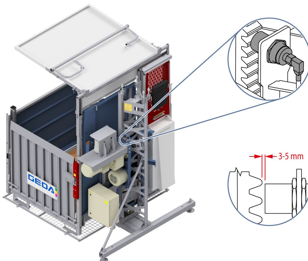
III. 56: Protection contre les dépassements et protection du câble
