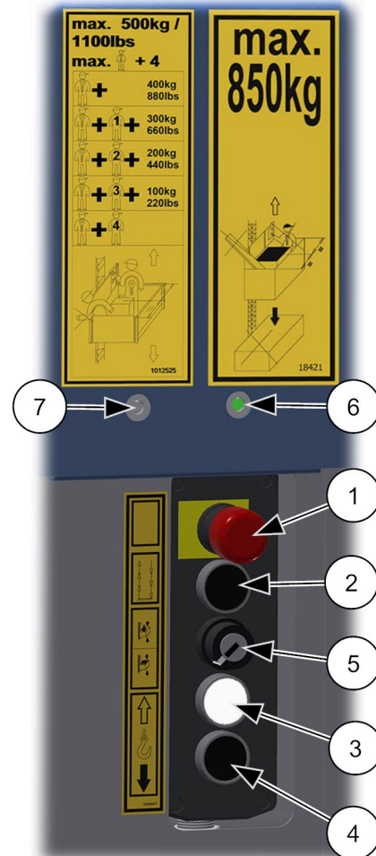
III. 41: Activer la commande extérieure
