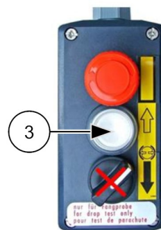
III. 66: Utilisation de la commande des essais de freinage
