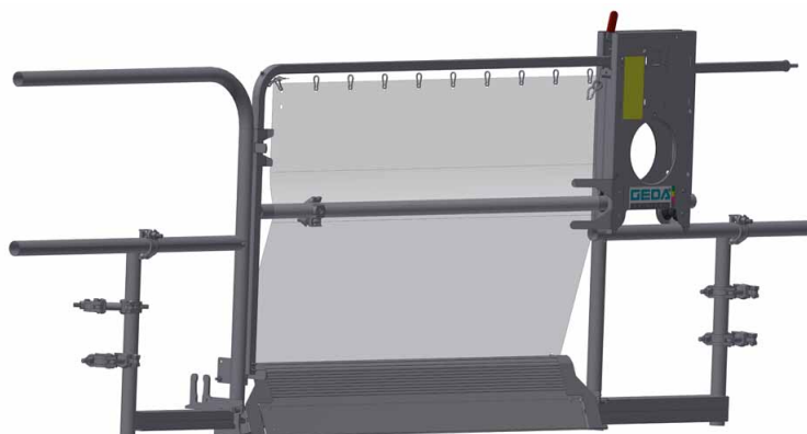
Ill. 38: Encagement d'accès sécurisé « Comfort » fermé (bâche)
