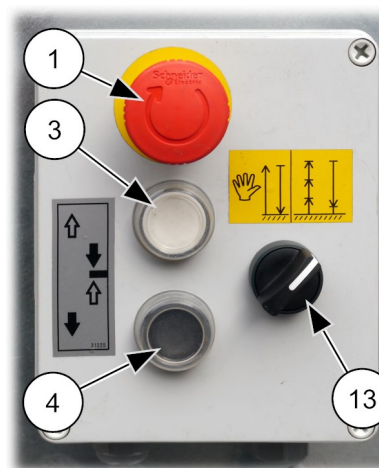
III. 45: Commande au sol pour le dispositif de protection (AUTOMATIQUE)
