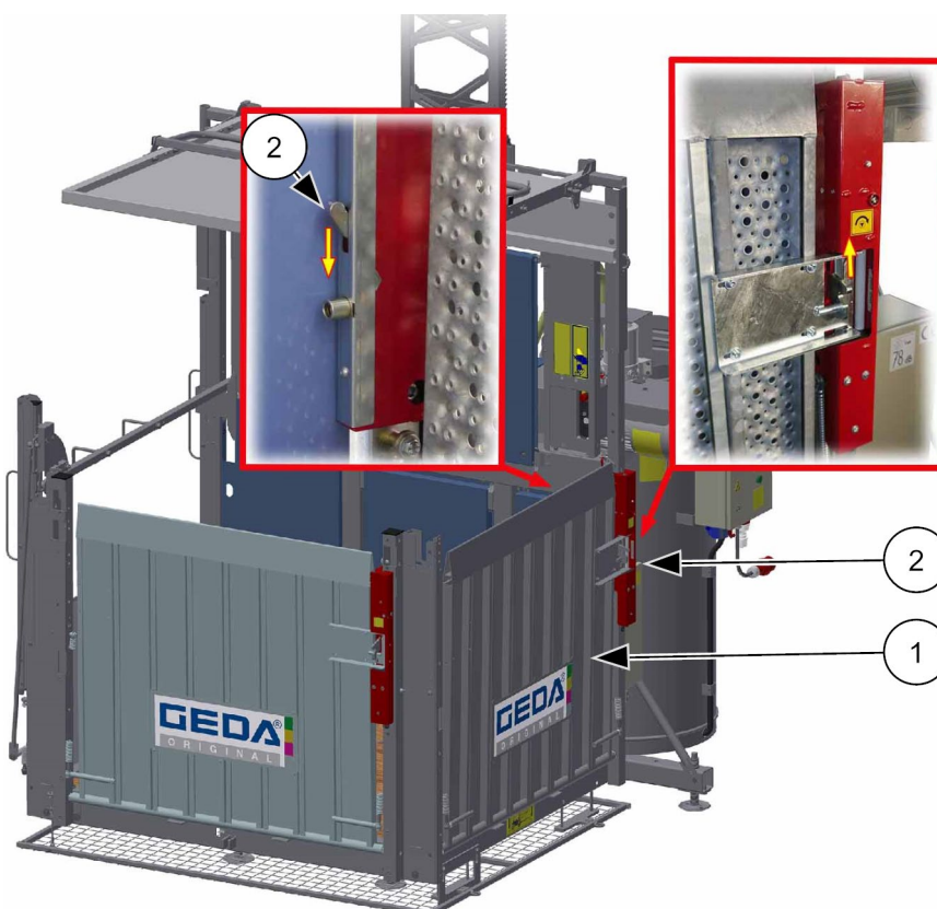
III. 26: Verrouillage Porte de chargement / Rampe
