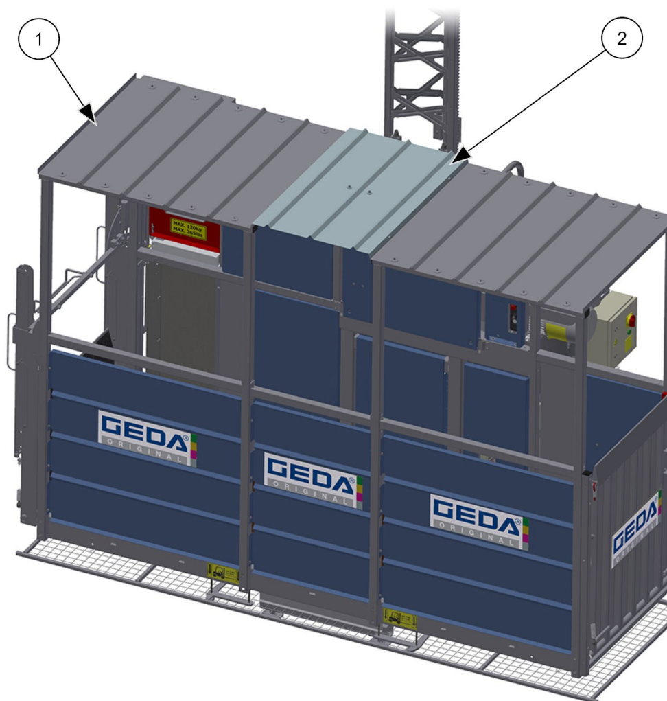
III. 54: Toit avec une ouverture de montage
