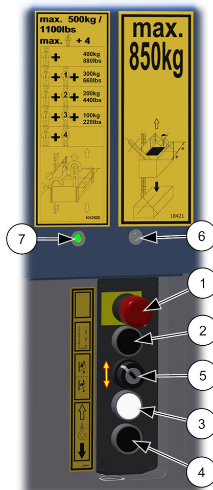
III. 71: Commande de la plateforme / utilisation de la plateforme de transport
