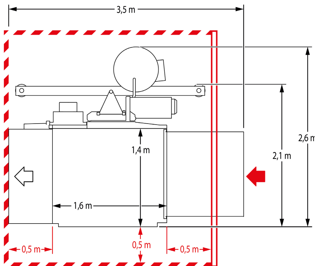
III. 5: Espace requis plateforme A
