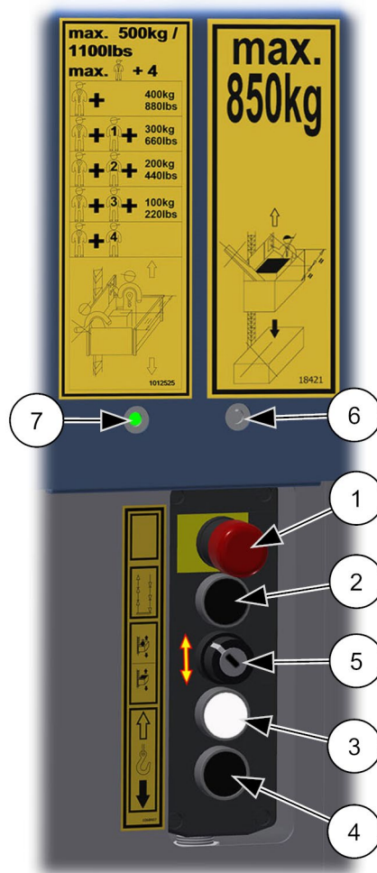
III. 47: Activer la commande de la plateforme
