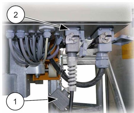
III. 68: Fiche isolante de la commande des essais de freinage
