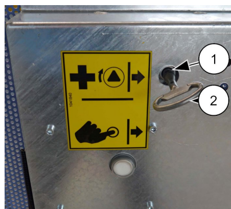
III. 23: Porte coulissante du déverrouillage d'urgence de l'extérieur
