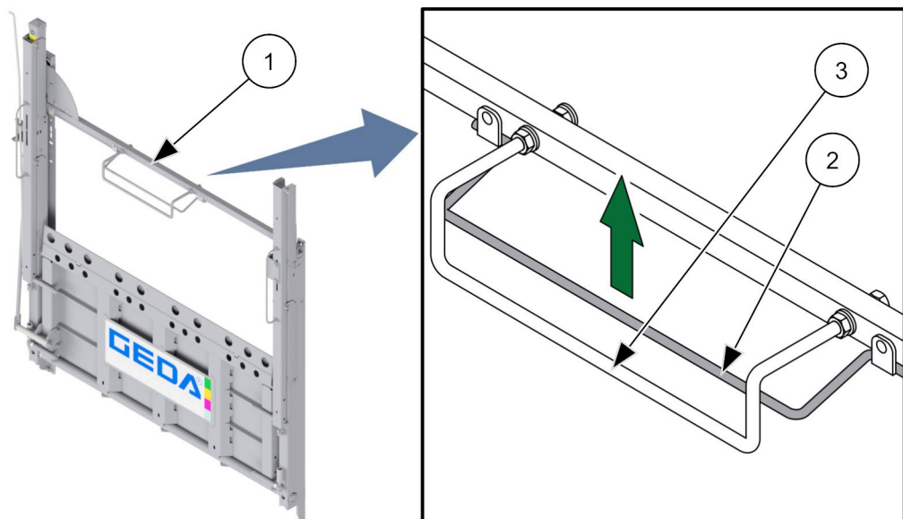
III. 31: Ouvrir la barrière avec verrouillage mécanique
