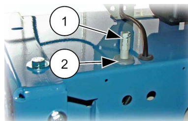
III. 72: Support du levier de desserrage du frein
