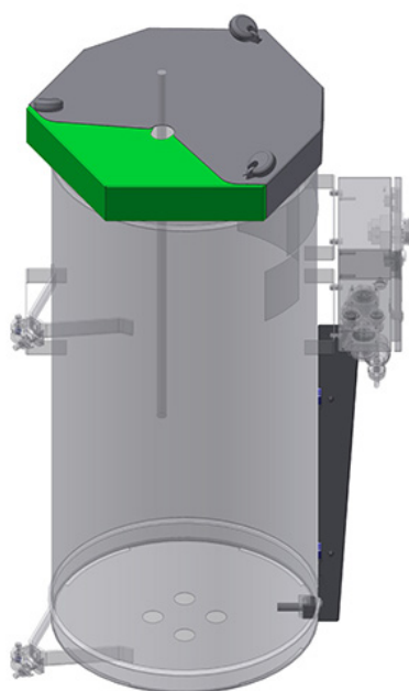
III. 61: Capot du réceptacle de câble
