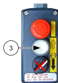
III. 69: Commande des essais de freinage
