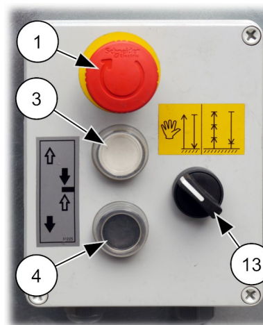
III. 43: Commande au sol pour le dispositif de protection (MANUEL)
