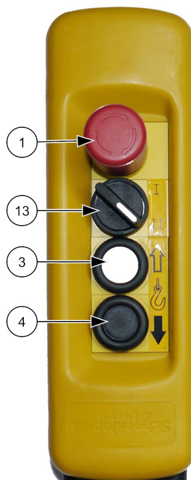
III. 44: Commande au sol / Commande manuelle (position II)
