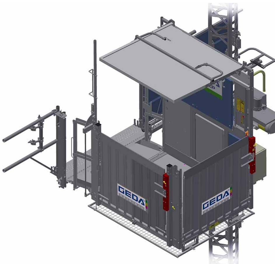
III. 30: Accès à la plateforme aux étages
