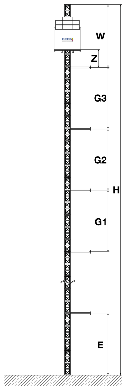
III. 3: Schéma Ancrage
