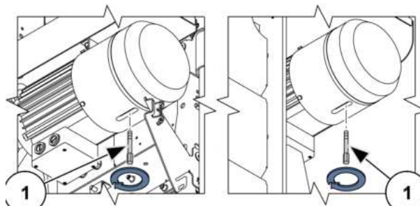
III. 109: Visser le levier de desserrage du frein dans les freins du moteur.
