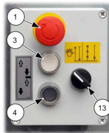
III. 77: Commande au sol pour le dispositif de protection (MANUEL)
