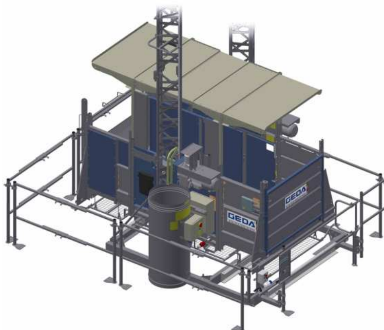
III. 38: Protection au sol de 1,10 m avec barrière
