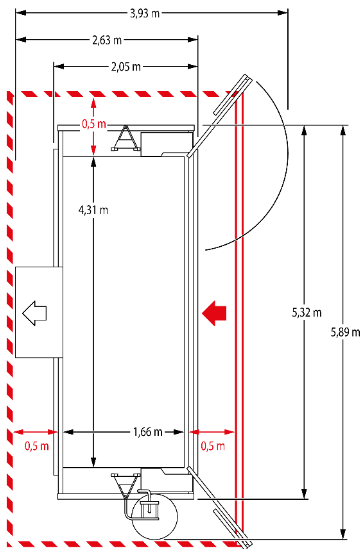
III. 33: Espace requis plateforme I
