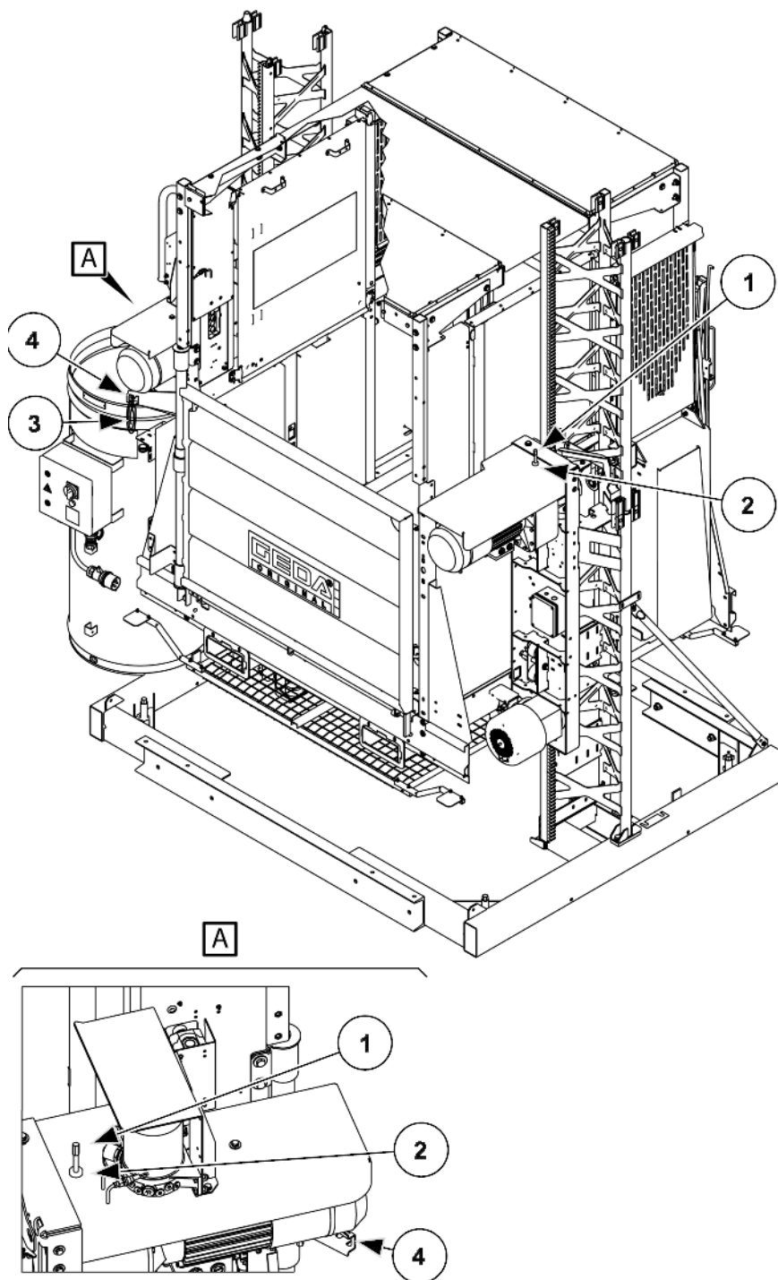
III. 106: Desserrage du câble du frein
