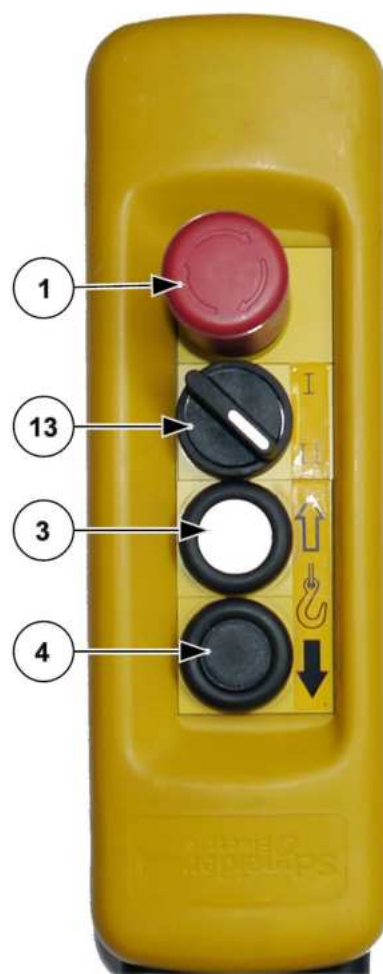
III. 78: Commande au sol / Commande manuelle (position II)
