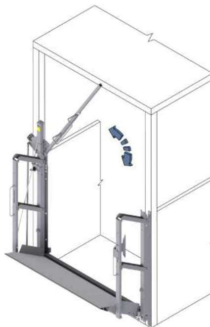
III. 54: Fermer la barrière avec verrouillage mécanique
