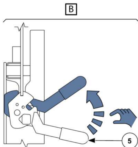
III. 61: Déverrouiller la rampe de chargement à entraînement électrique
