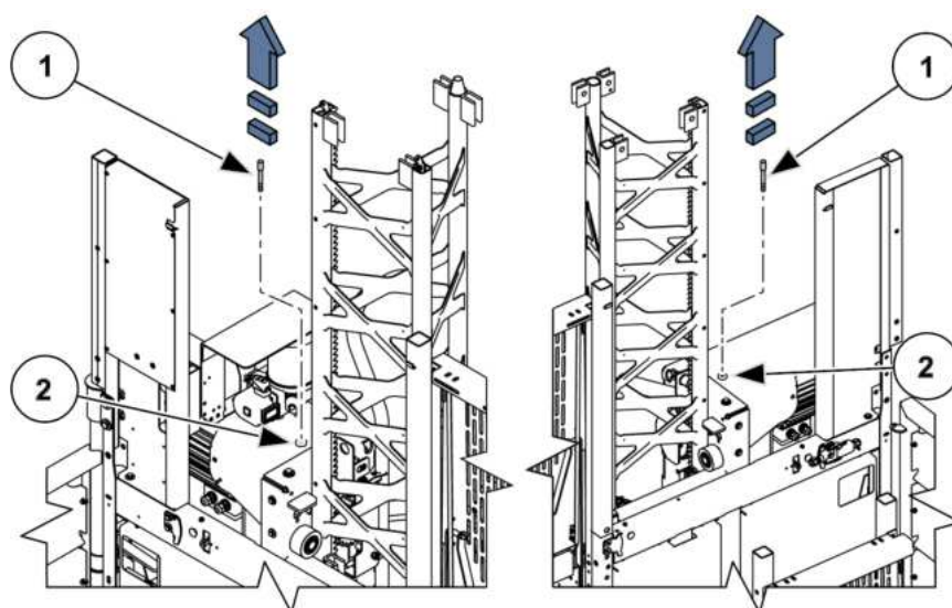
III. 108: Sortir le levier de desserrage du frein (1) du support (2)
