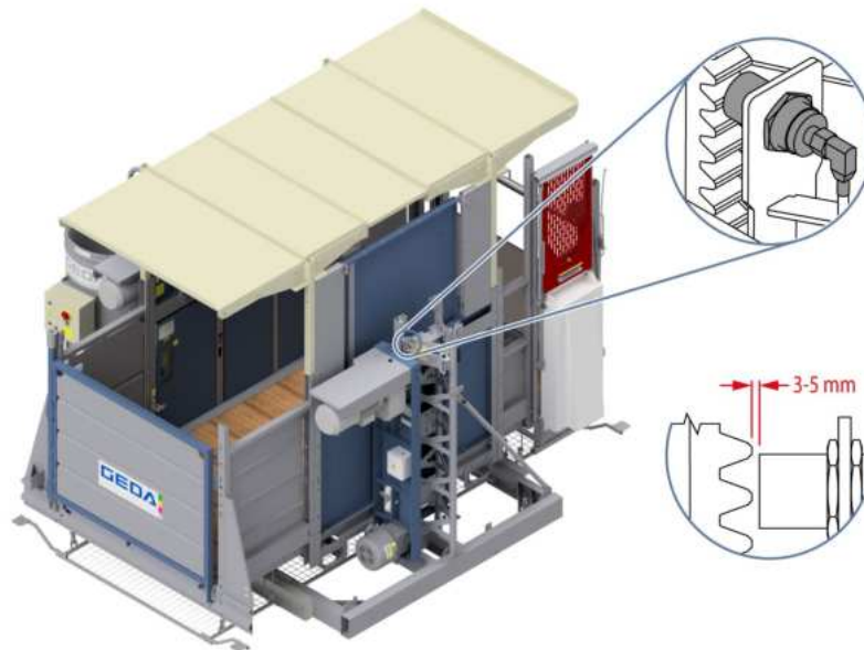
III. 90: Protection contre les dépassements et protection du câble
