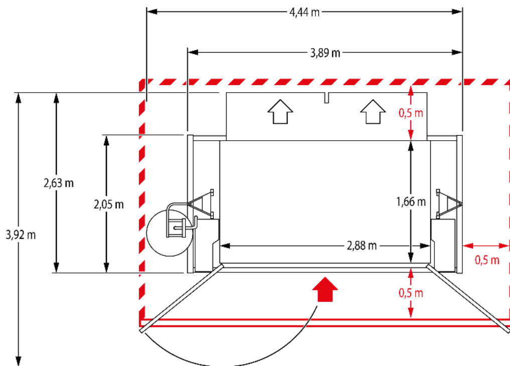
III. 21: Espace requis plateforme ED
