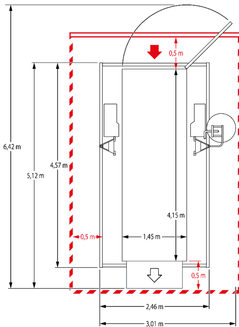
III. 9: Espace requis plateforme BL
