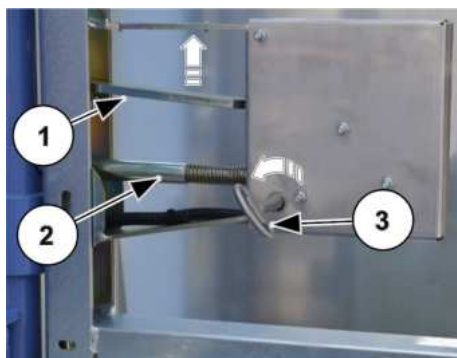
III. 48: Déverrouillage d'urgence de la rampe / Porte de chargement à l'extérieur
