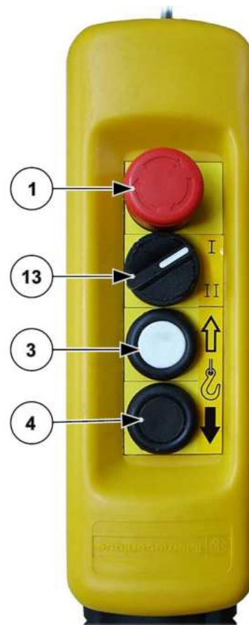
III. 76: Commande au sol / Commande manuelle (position I)
