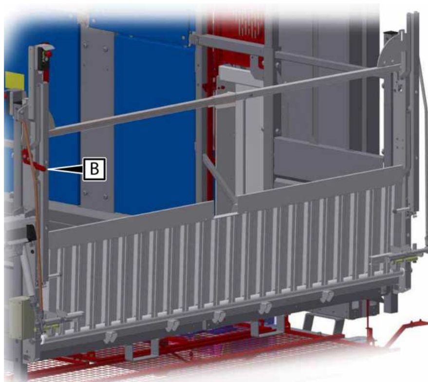
III. 60: Barrière électrique avec rampe de chargement de 2,82 m
