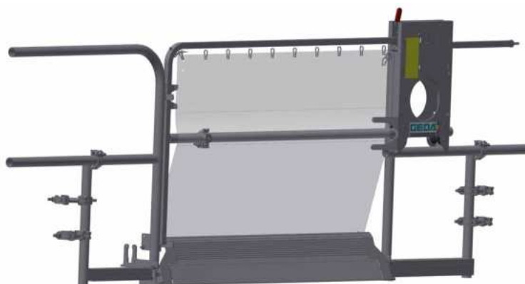
III. 67: Encagement d'accès sécurisé « Comfort » fermé (bâche)
