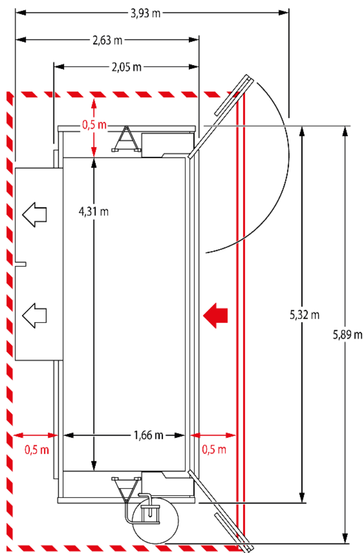
III. 29: Espace requis plateforme GD
