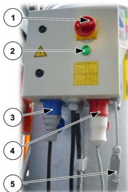
III. 34: Coffret de commande de la station au sol
