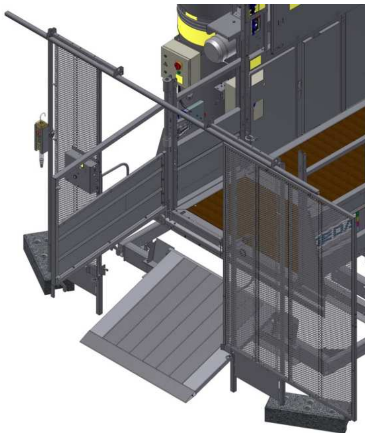
III. 43: Porte coulissante du dispositif de protection au sol ouverte
