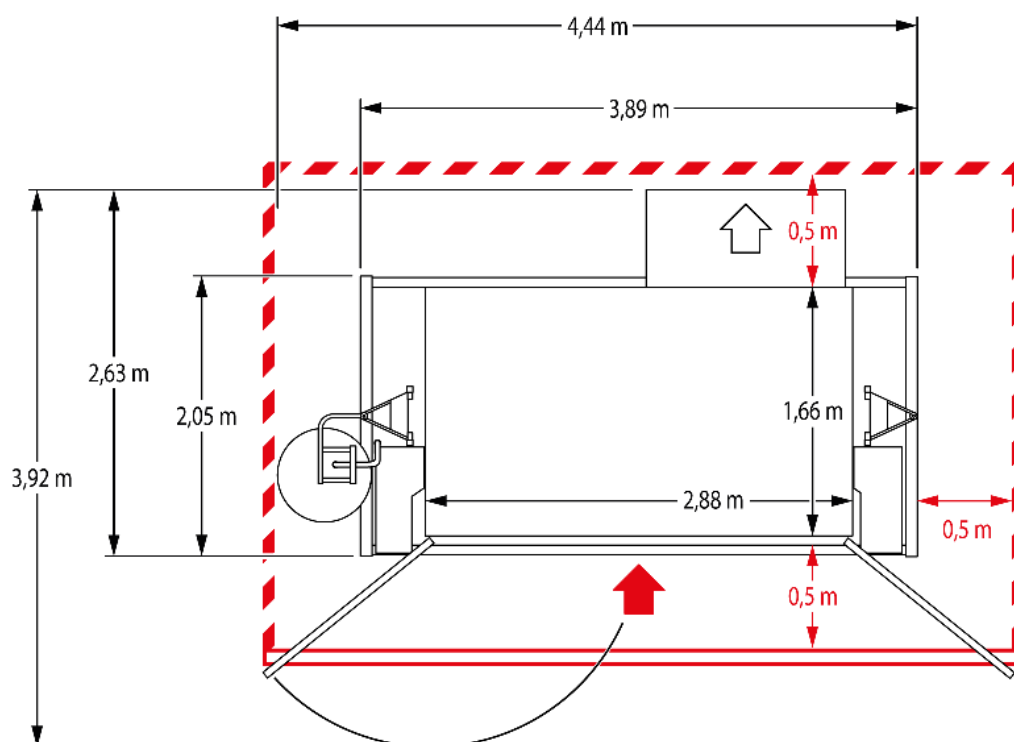
III. 17: Espace requis plateforme D
