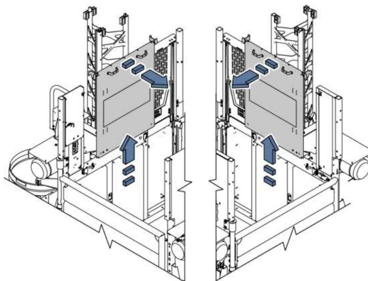
III. 107: Démonter la tôle de protection de montage
