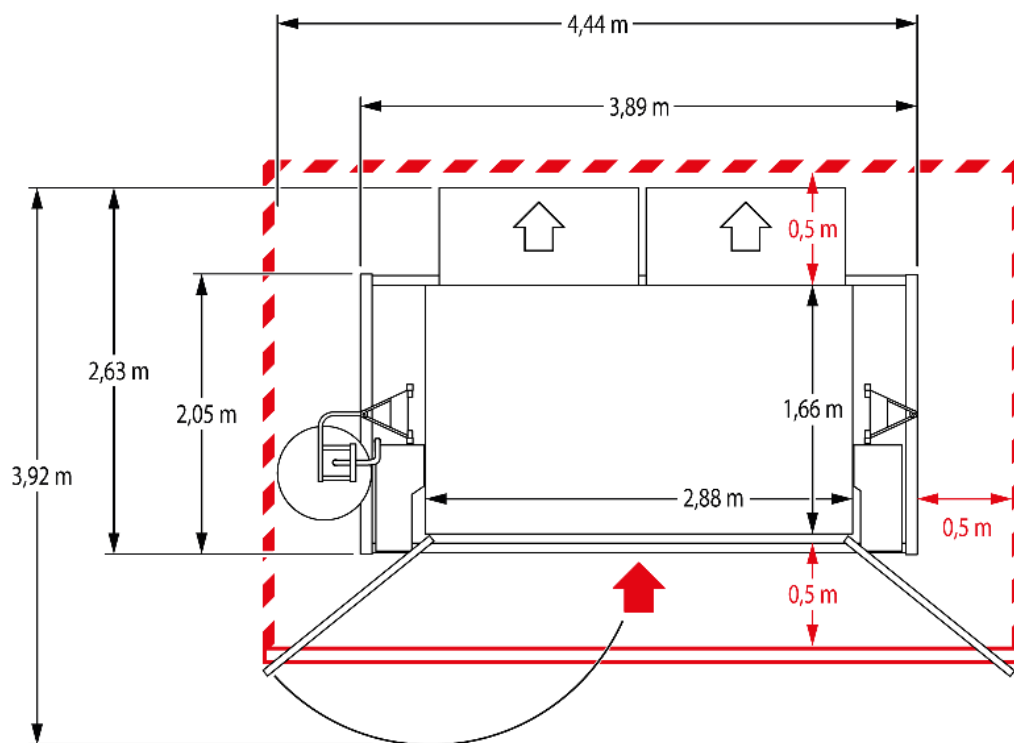
III. 19: Espace requis plateforme E
