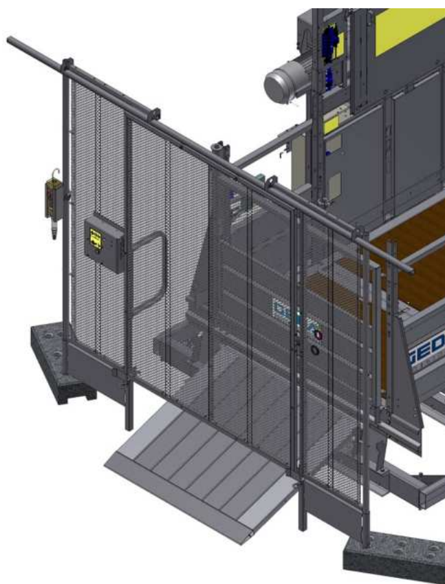
III. 39: Porte coulissante du dispositif de protection au sol fermée
