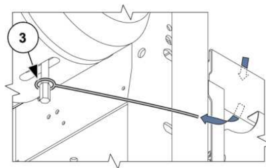
III. 112: Guidage du câble sans déflecteur
