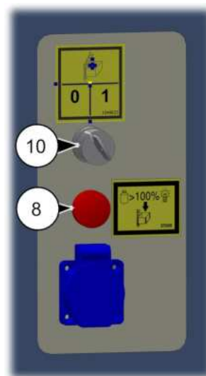
III. 35: Sélecteur Mode de fonctionnement Fonctionnement
