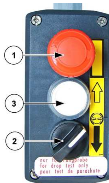
III. 84: Commande des essais de freinage
