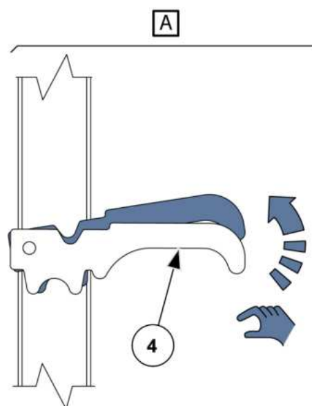
III. 59: Déverrouiller la rampe de chargement mécanique
