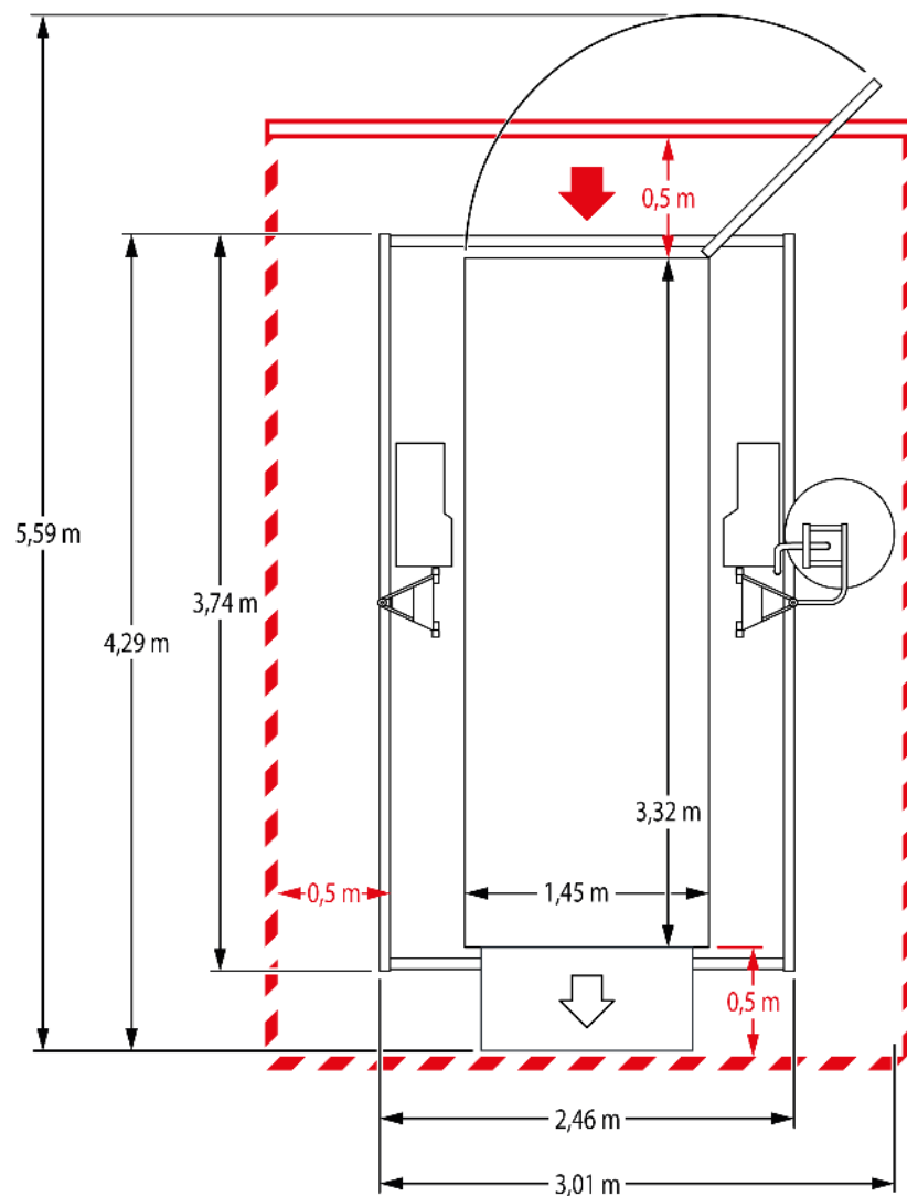
III. 13: Espace requis plateforme BS
