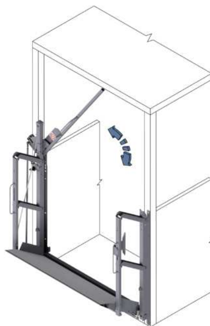
III. 56: Ouvrir/fermer la barrière avec verrouillage électromécanique
