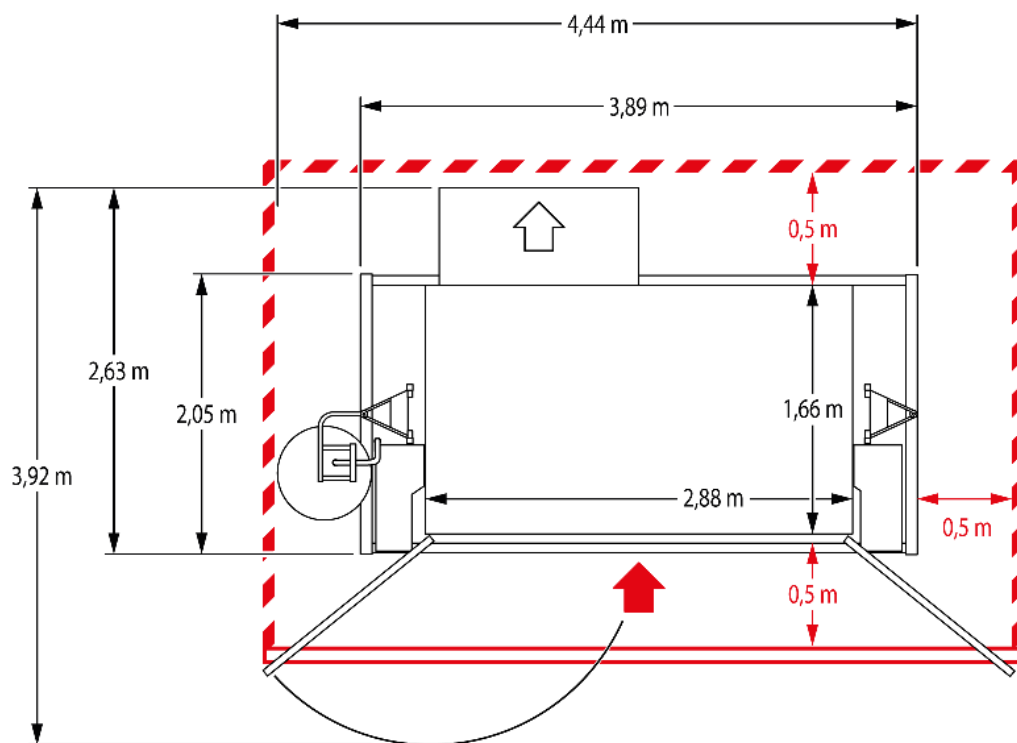
III. 15: Espace requis plateforme C
