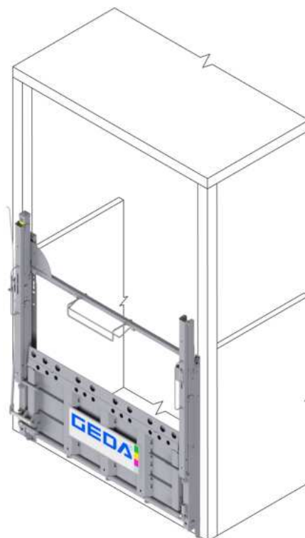
III. 52: Barrière avec verrouillage mécanique
