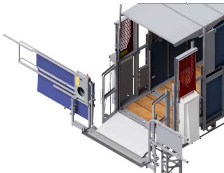
III. 51: Accès à la plateforme aux étages
