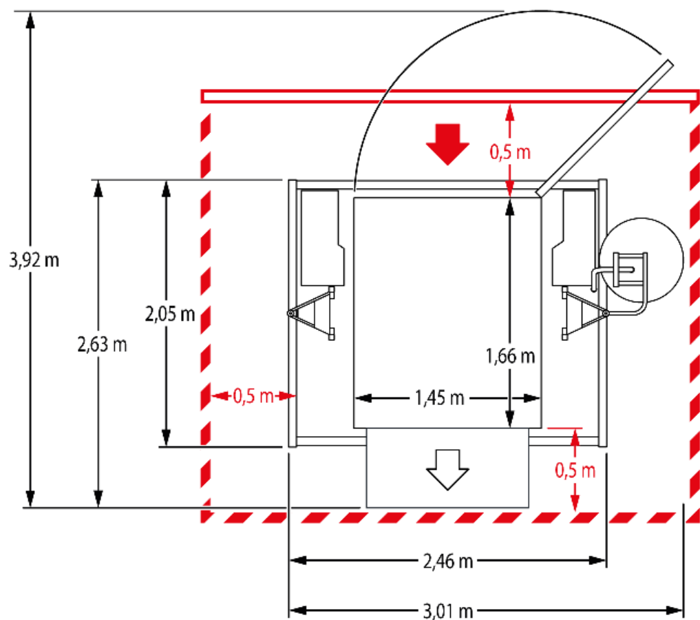
III. 5: Espace requis plateforme A
