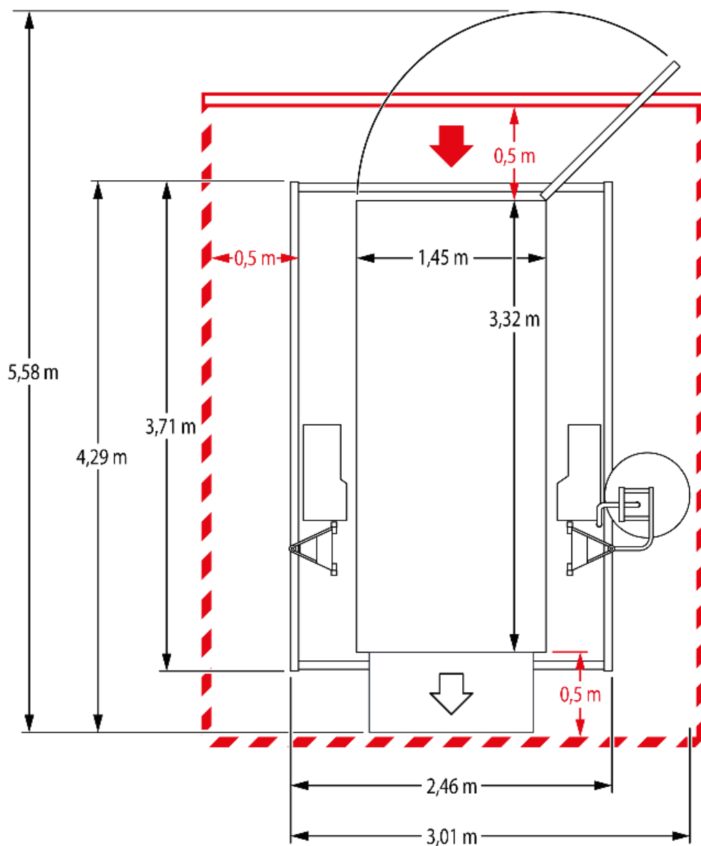
III. 7: Espace requis plateforme B
