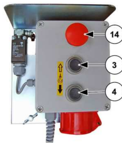
III. 80: Module électrique pour l'encagement d'accès sécurisé
