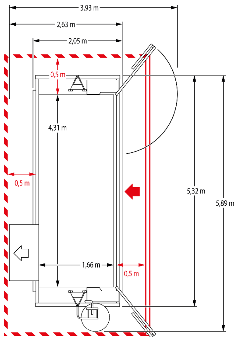
III. 25: Espace requis plateforme F
