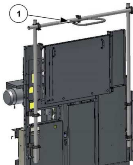
III. 94: Support individuel pour pièces d'échafaudage
