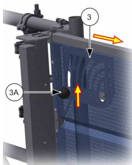
III. 73: Ouvrir/fermer l'encagement d'accès sécurisé « VARIO »
