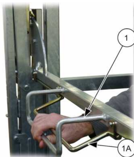
III. 53: Ouvrir la barrière avec verrouillage mécanique
