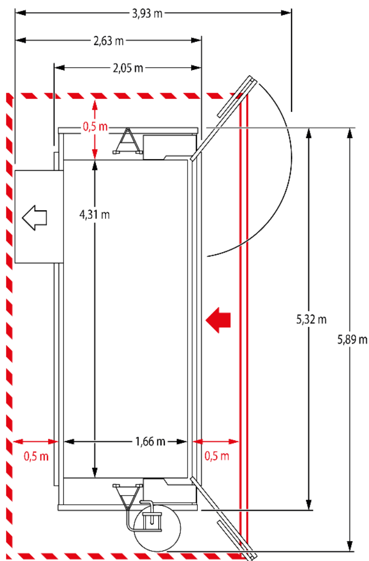
III. 27: Espace requis plateforme G
