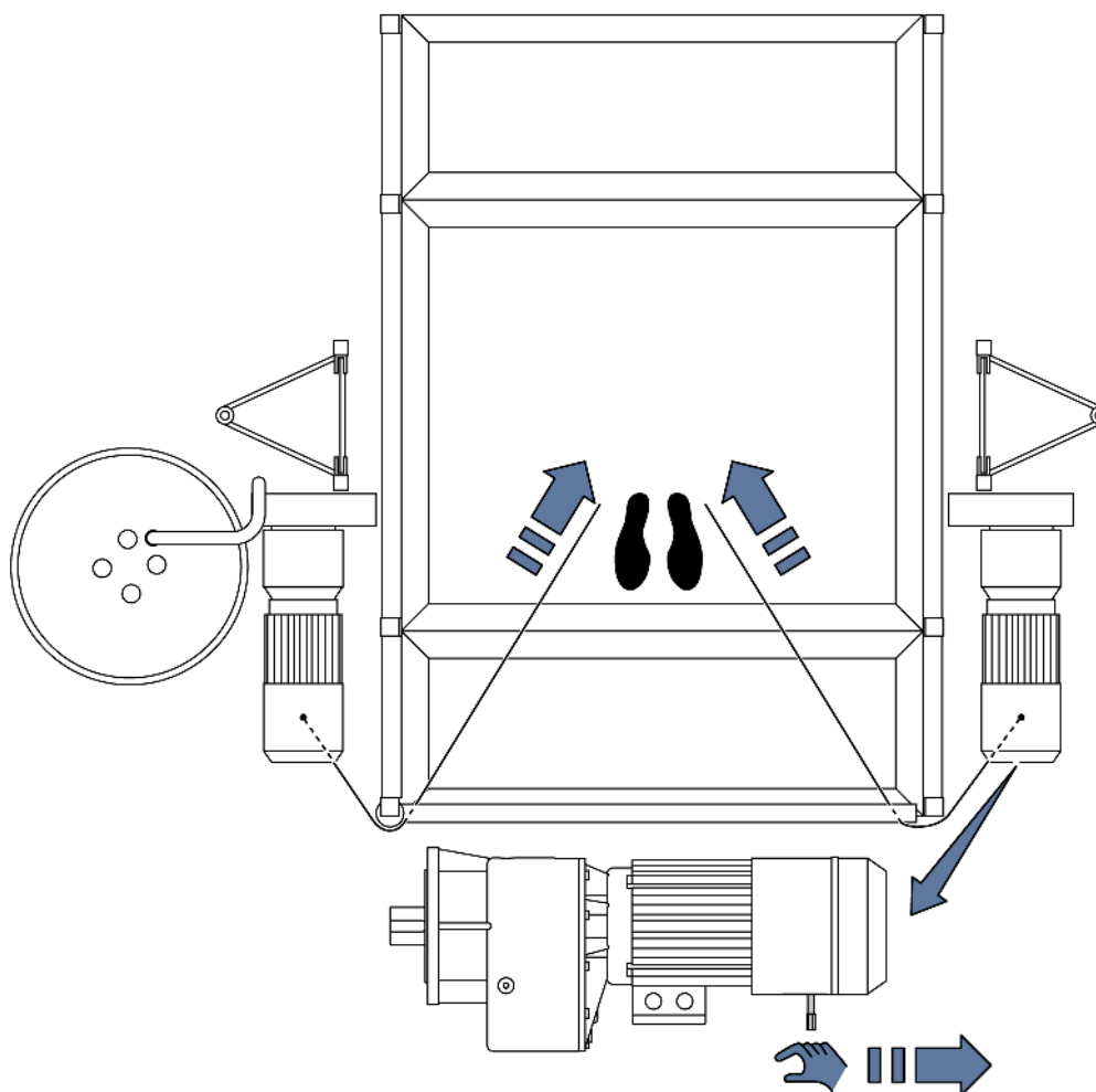
III. 113: Déclencher l'abaissement d'urgence sans le déflecteur !
