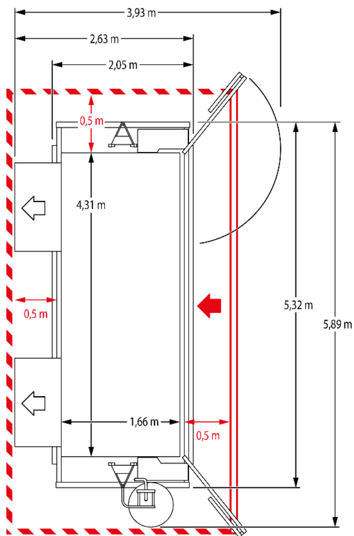
III. 31: Espace requis plateforme H
