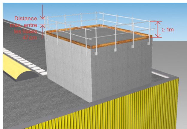
17 Garde-corps périphérique solidement ancré au bâtiment, puits de lumière résistant à la rupture.
