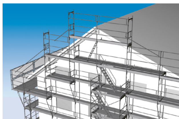
1 Protection collective durant la phase de construction
