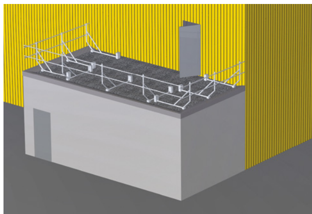
18 Balustrade librement implantée, posée avec contrepoids (solution alternative).
