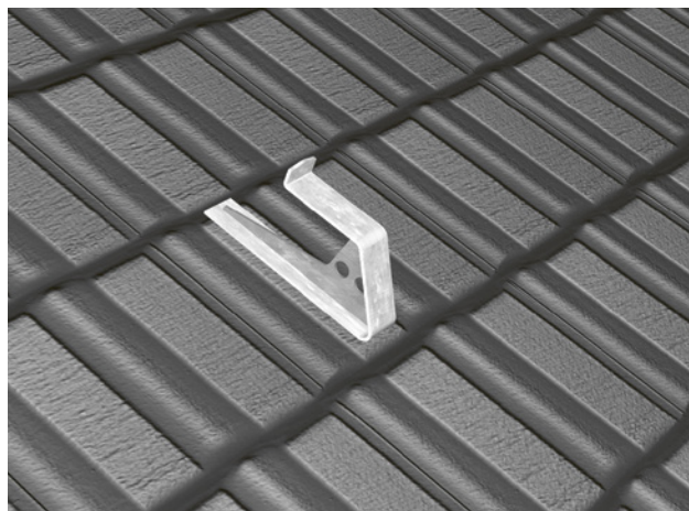
15 Crochet de sécurité en toiture conforme à la norme SN EN 517
