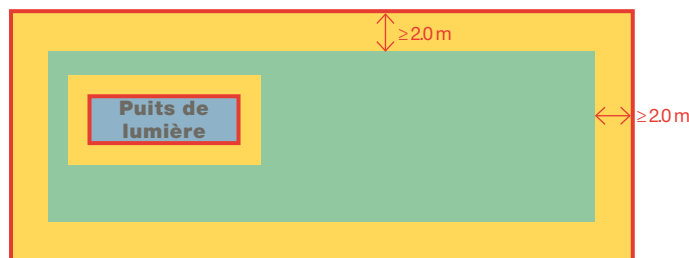
23 Zones dangereuses sur un toit plat.
