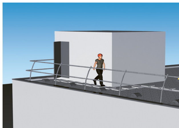
2 Protection collective durant la phase d'utilisation
