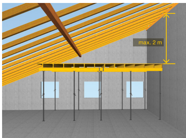
11 Échafaudage de retenue sous une structure porteuse
