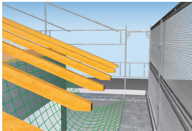
12 Solution avec filet de sécurité dans le débord de toit
