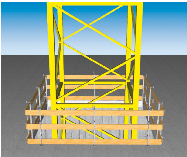
21 Garde-corps périphérique en trois parties autour d'une trémie dans la dalle.
