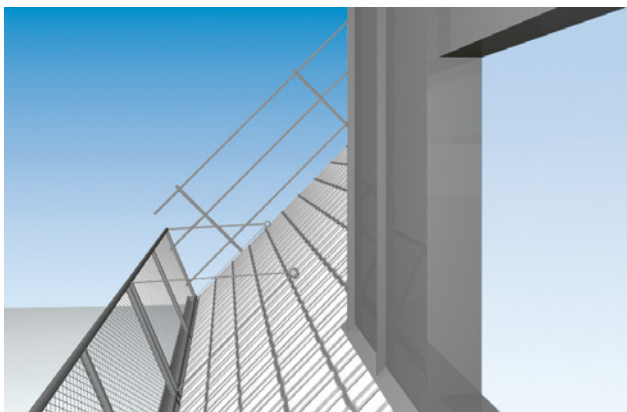
5 Paroi de retenue sur le toit inappropriée pour les travaux sur les lucarnes.
