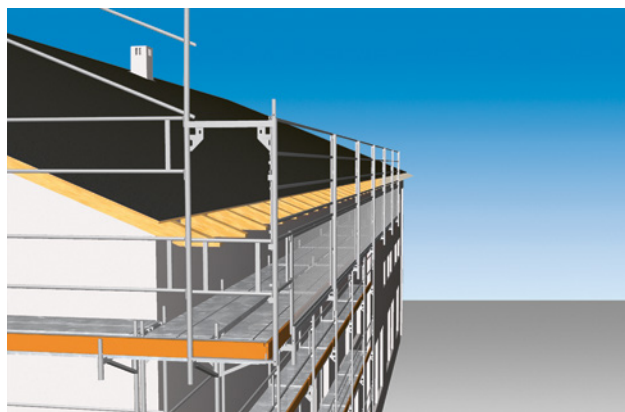
13 Solution avec console intérieure sur l'échafaudage Celle-ci permet d'empêcher la chute de personnes entre l'échafaudage et la maçonnerie.
