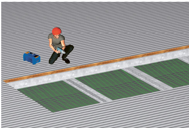
19 Filet de sécurité sous une ouverture en toiture.
