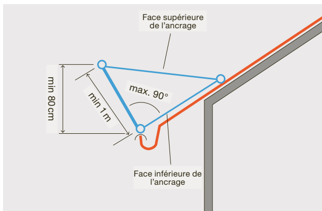
4 Dimensions de la paroi de retenue sur le toit
