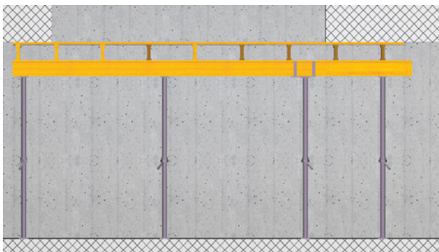
20 Ouverture dans une dalle de toiture fermée par un échafaudage de retenue.
