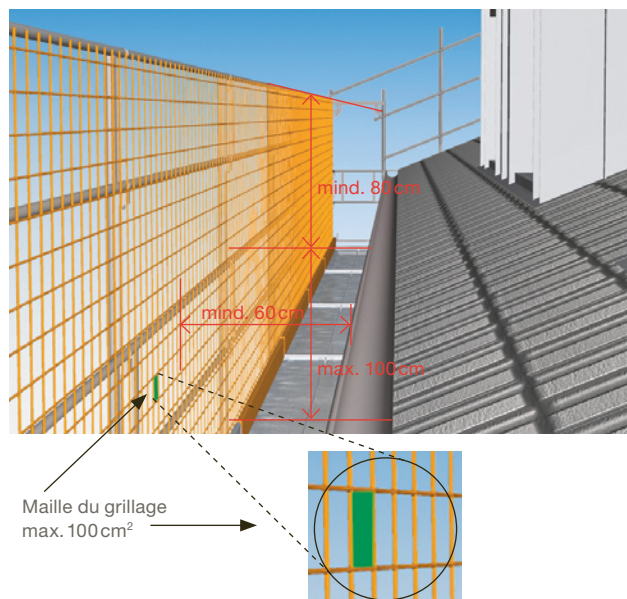
3 Pont de ferblantier avec paroi de protection de couvreur, variante avec un grillage sur toute la hauteur
