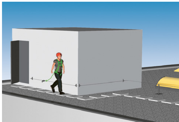
24 Accès sûr pour des travaux de courte durée sur un toit plat.
