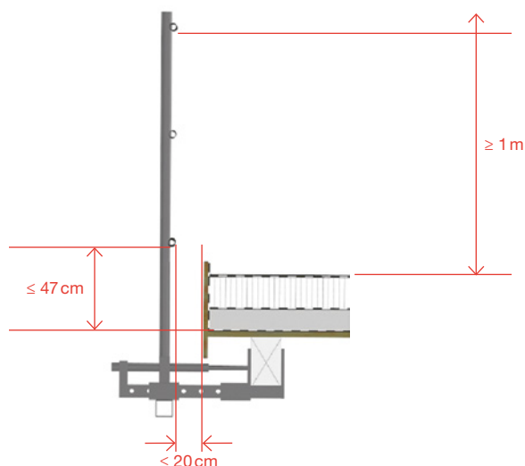
8 Garde-corps périphérique du côté des pignons (coupe transversale) avec tube supplémentaire pour isolations d'épaisseur importante.
