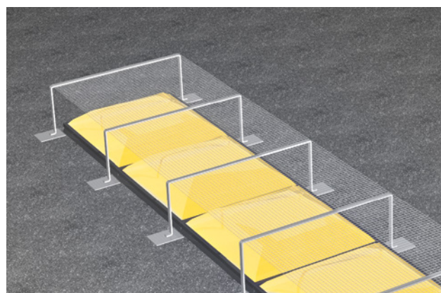
22 Puits de lumière en matière synthétique avec protection collective (grillage).
