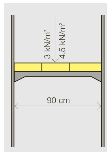
Figure 3: échafaudage pour travaux de maçonnerie ou de taille de pierres
