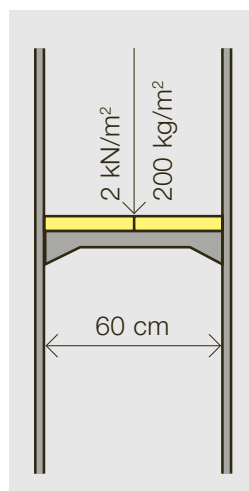
Figure 2: échafaudage pour travaux de crépissage ou de peinture
