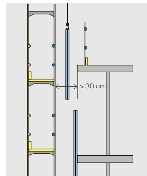
Figure 13: mise en place d'éléments de façade
