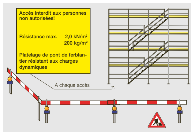
Figure 4: la charge utile des échafaudages de service doit être clairement indiquée sur un panneau à chaque accès.
