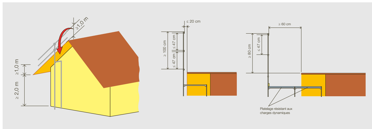
Figure 22: garde-corps périphérique du côté des pignons
