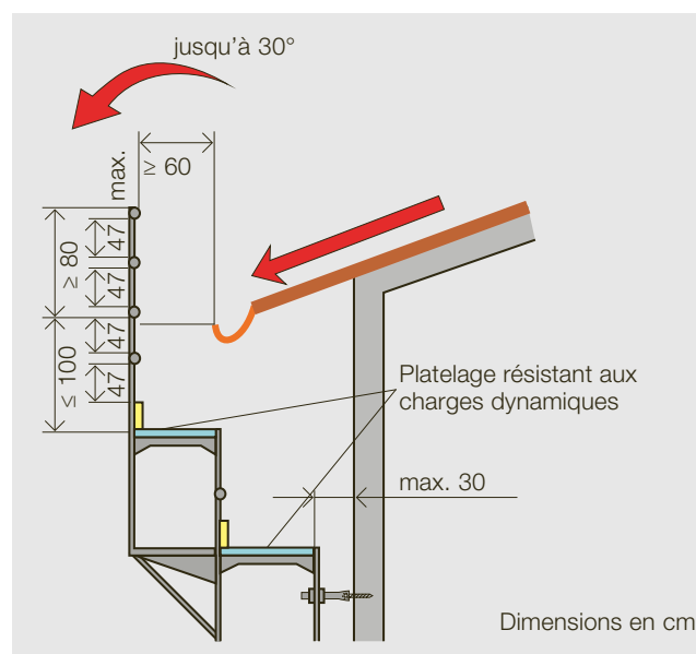
Figure 20: garde-corps périphérique d'un pont de ferblantier pour un toit de pente \geq 30^\circ
