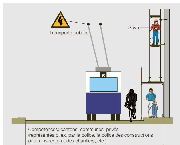
Figure 2: interface entre le chantier et les voies publiques. Les mesures nécessaires sont prises d'un commun accord avec les autorités compétentes.
