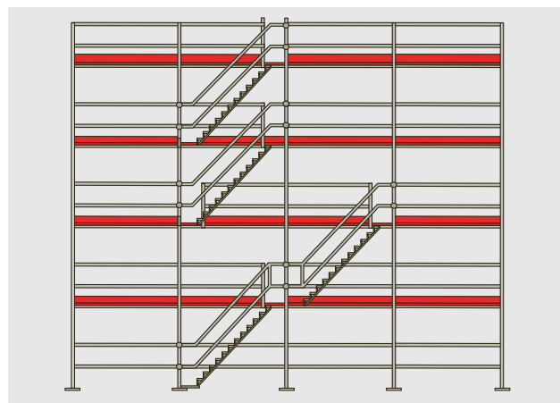
Figure 15: accès sûr: escaliers avec paliers
