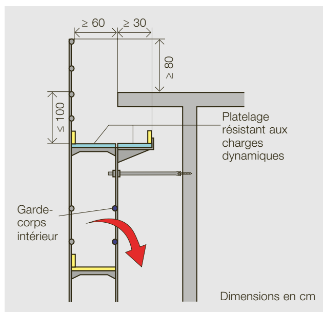
Figure 18: pont de ferblantier
